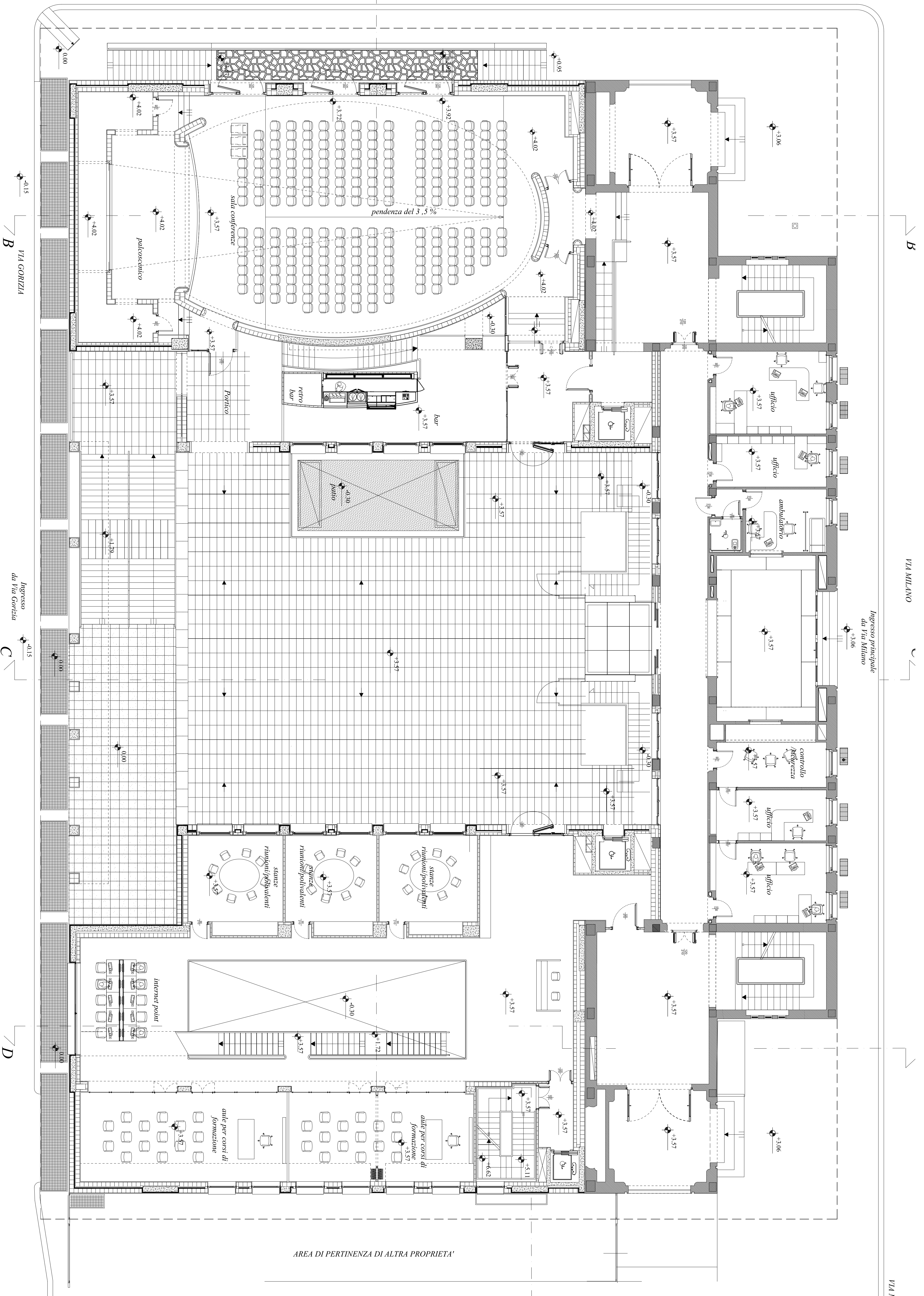
PIANTA PIANO TERRA - quota +3.75 m (circa 1450 mq) scala 1:100
